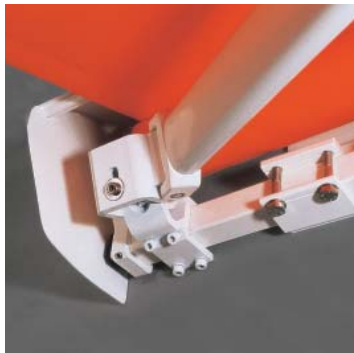
Armkonsole
